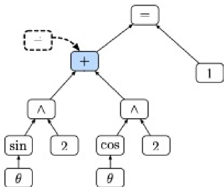
Replace Node
